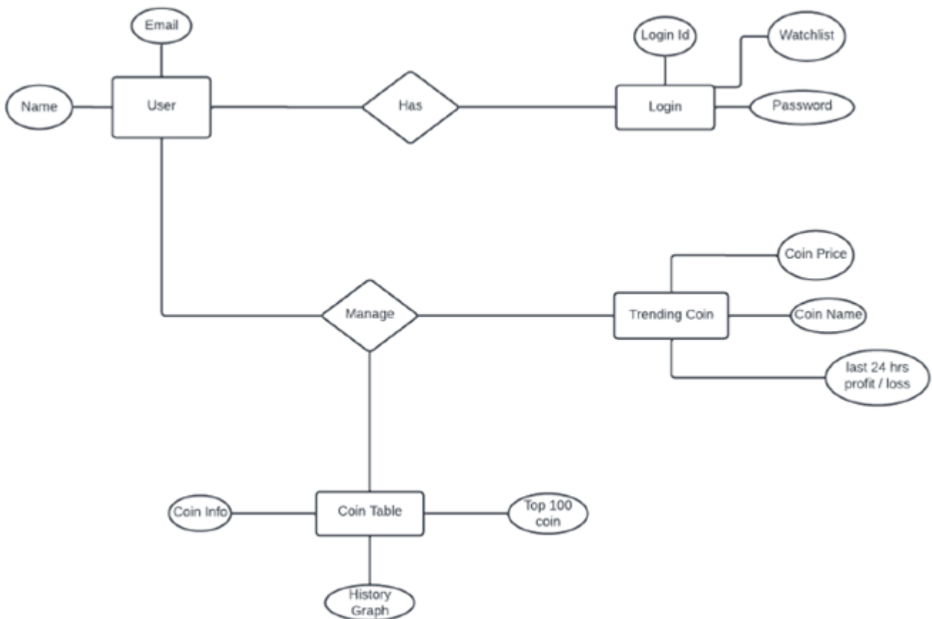
Fig. 1. ER Diagram
